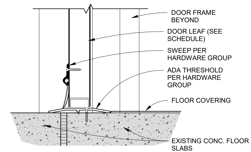
DETAIL@ HOLLOW METAL DOOR SILL
