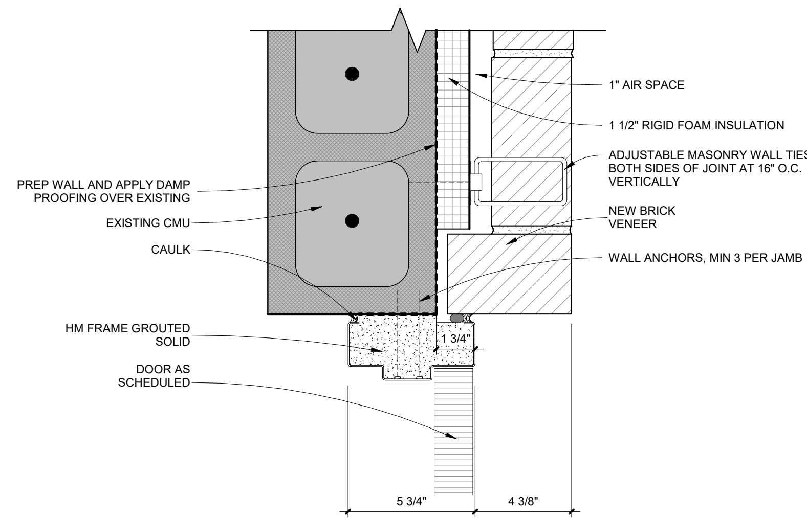
PLAN DETAIL@ HOLLOW METAL DOOR JAMB
